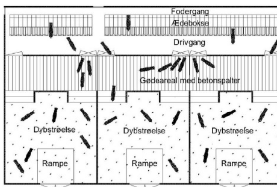
Figur 8.11. Tv.: Eksempel på indretning af løbestald med dybstrøelse og spaltegulv til løsgående søer. Th.: Plantegegning af stald med dybstrøelse og spaltegulv til løsgående drægtige søer (Foto: Sommer et al. , 2006).
