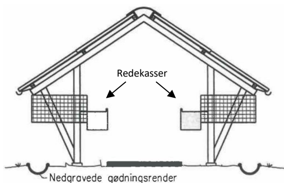
Figur 8.33. Tv.: Snittegning af minkhal med bure i to rækker og nedgravede gødningsrender (Kilde: Landbrugets byggeblade gr.nr. 110.5-02/1997). Th.: Foto af nedgravede gødningsrender (Kilde: M.H. Hansen, Brønderslev kommune). Viste anordninger for afledning af drikkevandsspild udenom gødningsrenderne er ikke lovpligtige.
