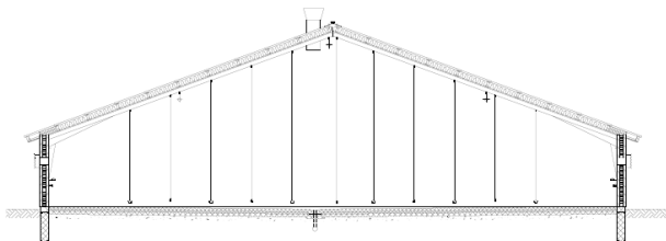
Figur 8.30. Tværsnit af en stald (gulvsystem) til hønnikeopdræt (Tegning: SEGES).
