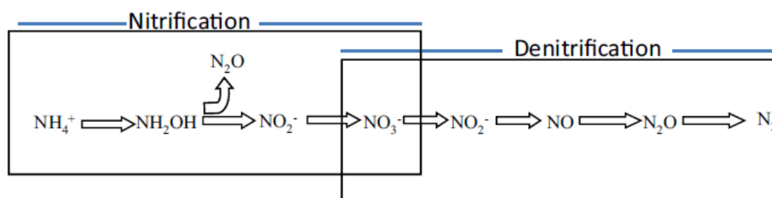
Figur 8.1. Skematisk præsentation af nitrifikations- og denitrifikationsprocesserne, hvorunder NH_4^+ først omdannes til nitrit og nitrat og derefter reduceres til frit kvælstof (Chatwick et al., 2011).
